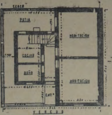
PLANTA BAJA
